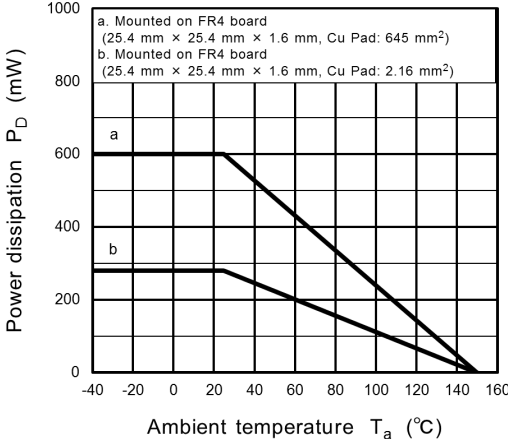
Fig. 7.13 P_D - T_a
