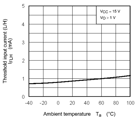
Fig. 12.2.4 I_{FLH} - T_a
