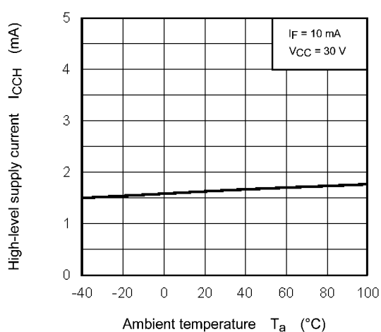
Fig. 12.2.6 I_{CCH} - T_a
