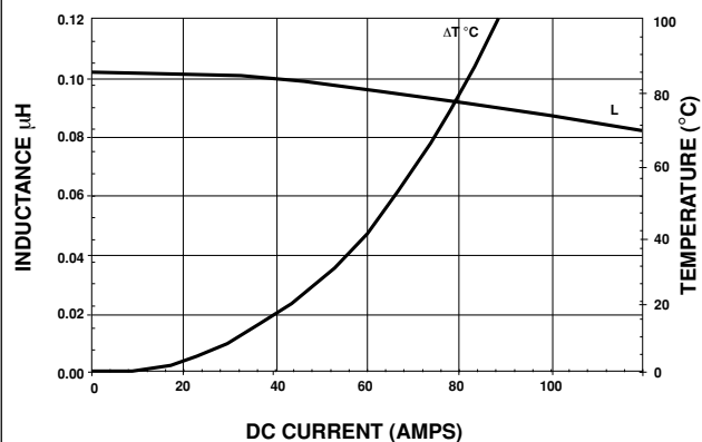
IHLP-5050EZ-01 0.10 \mu H
