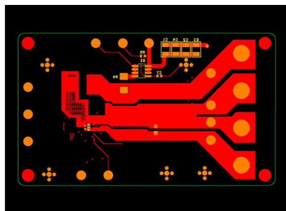
Figure 17. Bottom Layer
