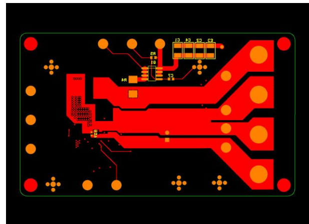
Figure 17. Bottom Layer
