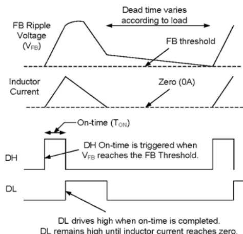
Fig. 6 - Power-Save Mode
