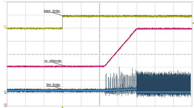
Fig. 30 - Prebias Start Up
