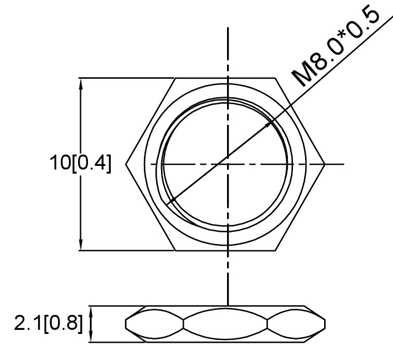
NUT
