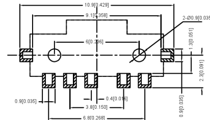
PCB板位置尺寸
