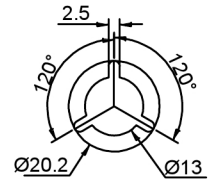
DETAL:A SC 10:1
