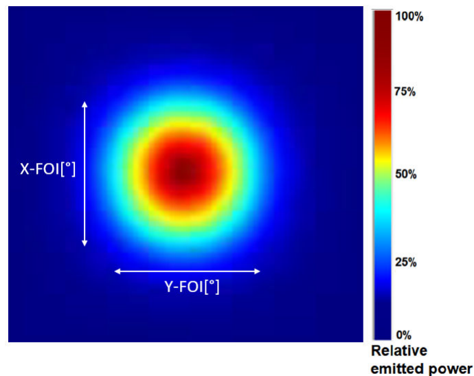
Figure 28. VL53L4ED FoI
