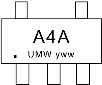
SOT23-5/SC70-5
