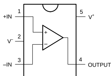
SOT-23 的 - LMV611
