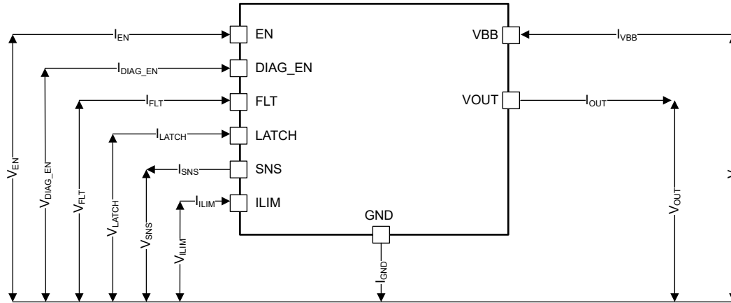
Figure 6-1. Parameter Definitions
