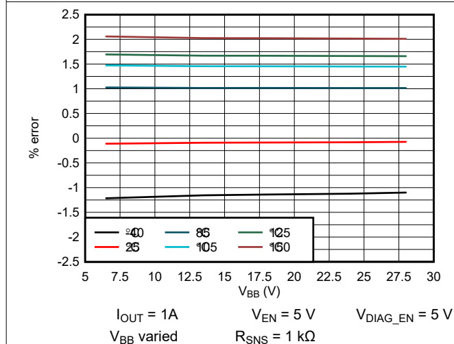
Figure 5-11. K_{SNS} Error vs V_{BB}
