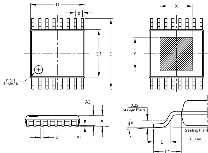
TSSOP-16EP
