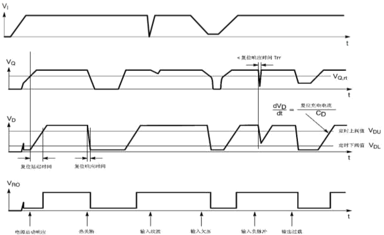
图 3 复位时序图
