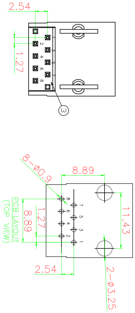
网络插座外形图
