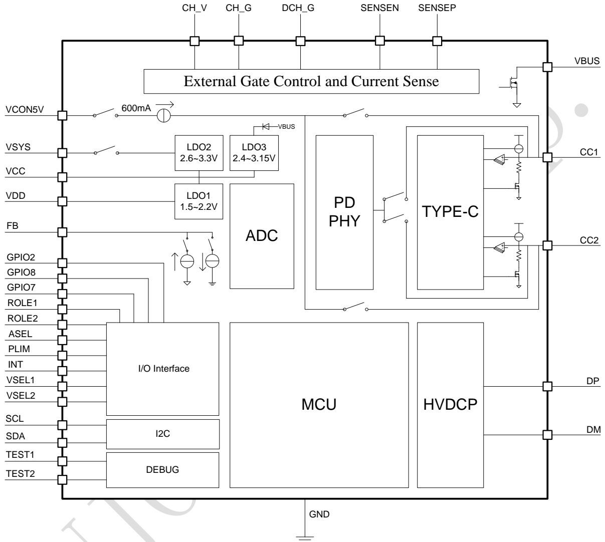
图 1. IP2716T 结构框图
