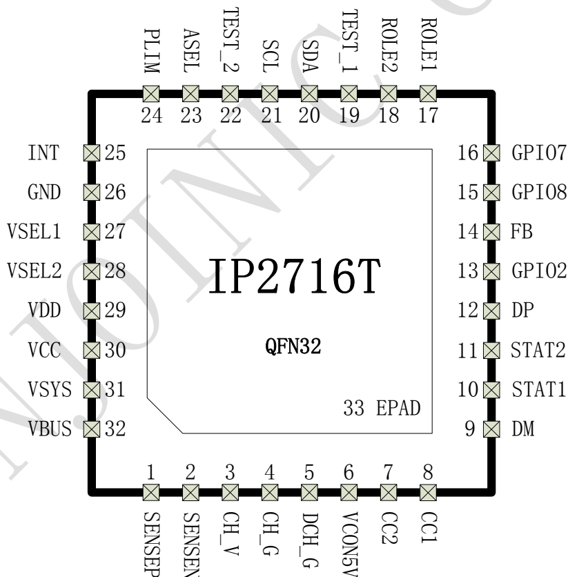
图 7. IP2716T 引脚图 (顶面图)
