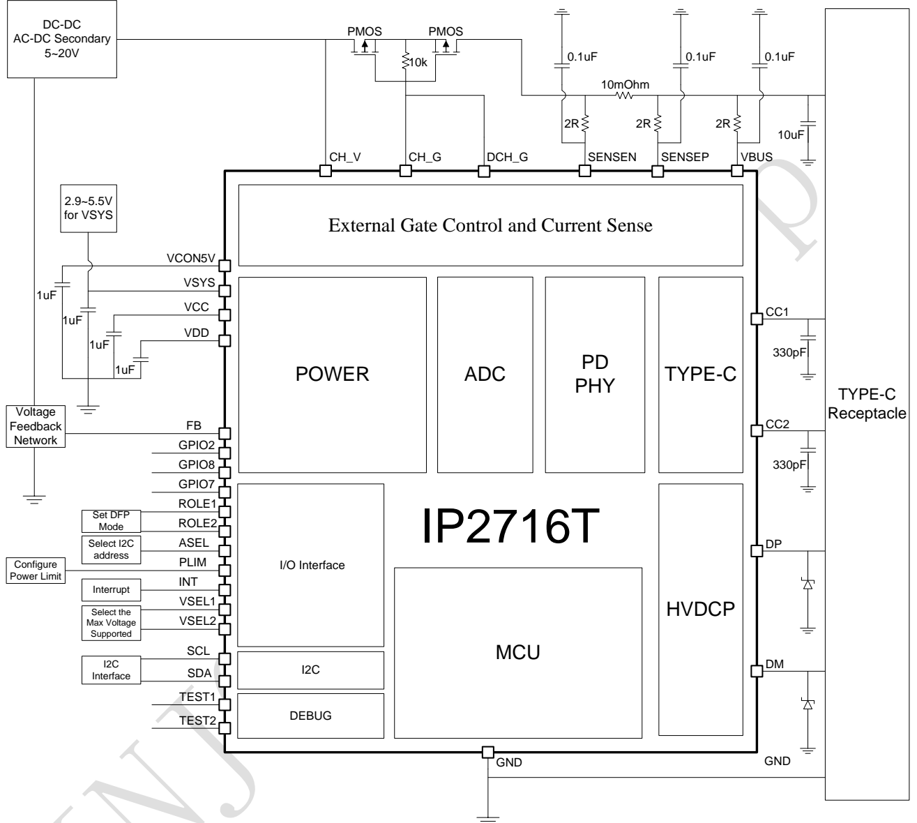
图 3. 电源适配器应用图
