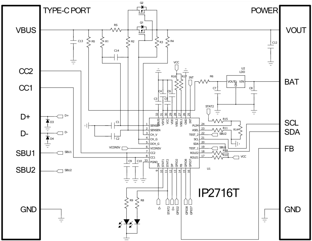
图 6 为 IP2716T 移动电源应用原理图，配置 DRP 模式，最大支持 20V 电压。
