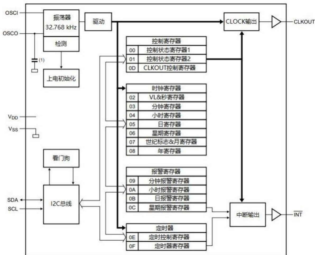
图 2. PCF85163 方框图
