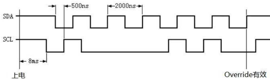
图 4. Override 时序图
