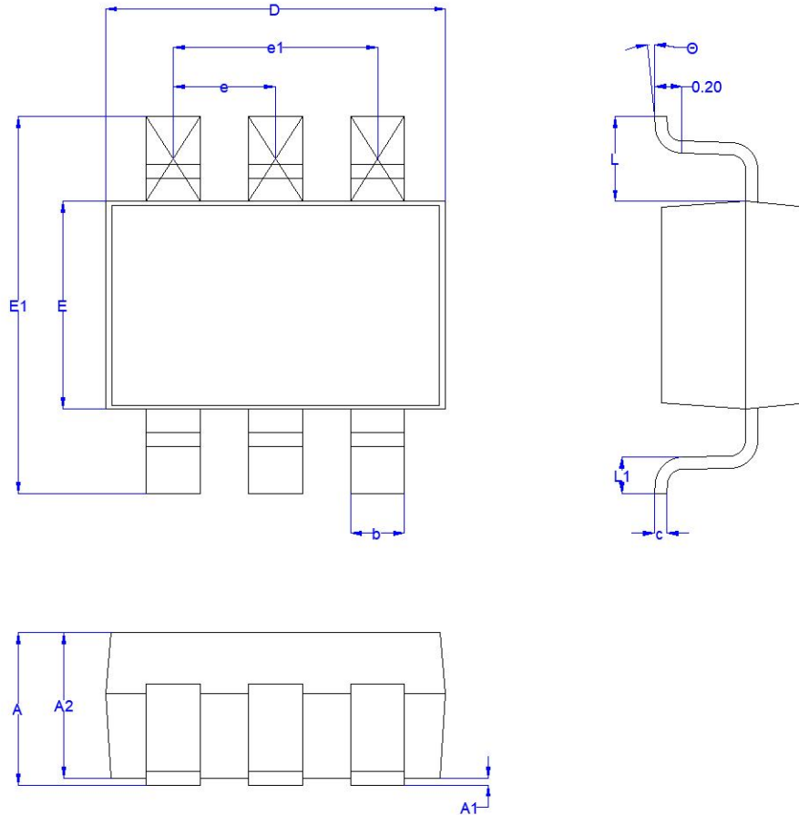
SOT-363(MicroPak-6)
