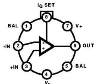
ICL7611, ICL7612 (METAL CAN) TOP VIEW
