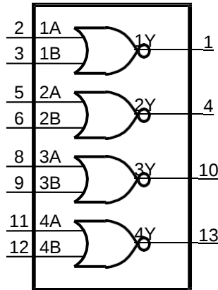
图 1 逻辑符号
