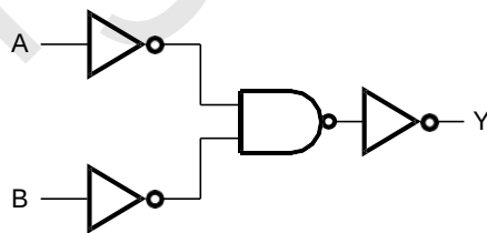
图 3 逻辑框图
