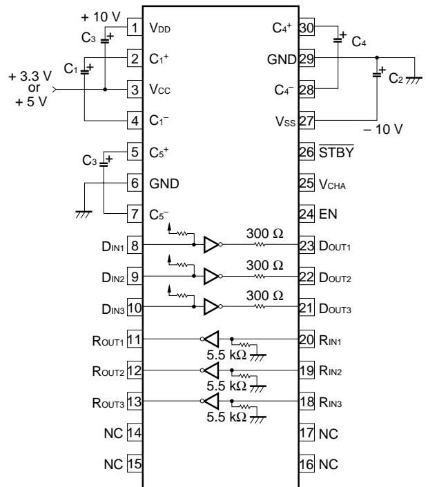
μPD4723
