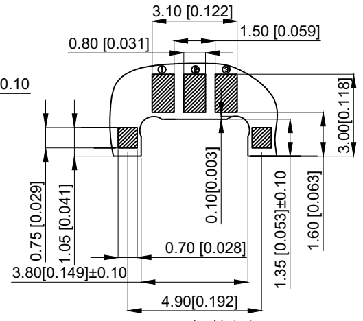
PCB. 安装图
