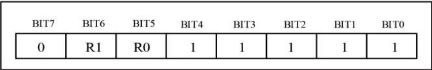
图 2-6 配置寄存器
