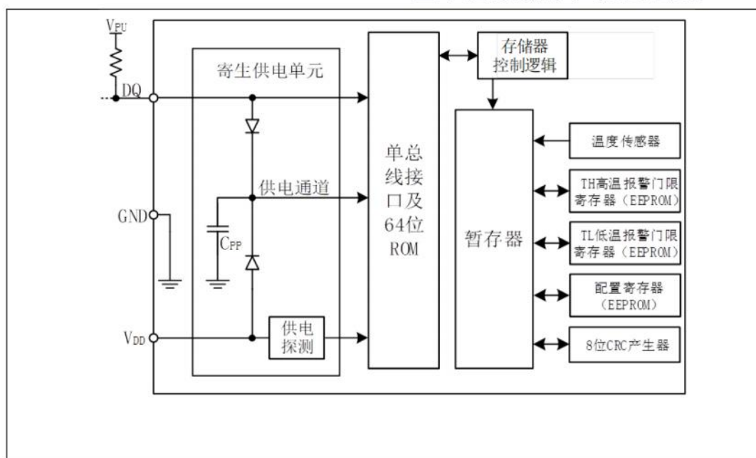
图 2-1 产品功能框图
