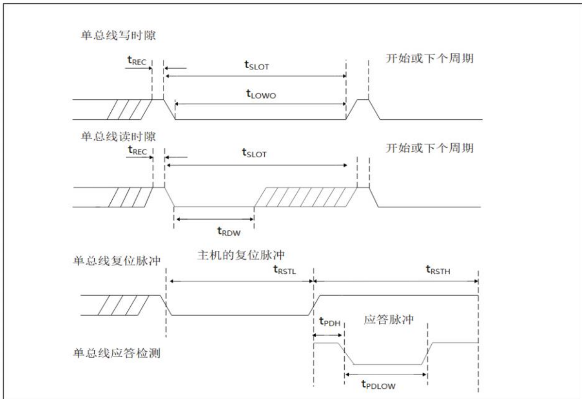
图 1-2 时序图
