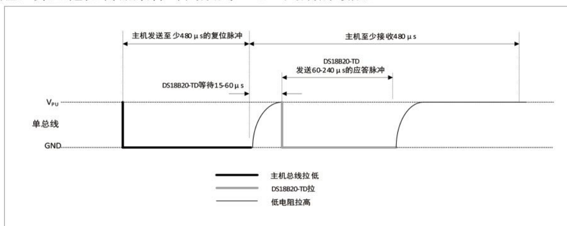
图 2-11 初始化序列时序
