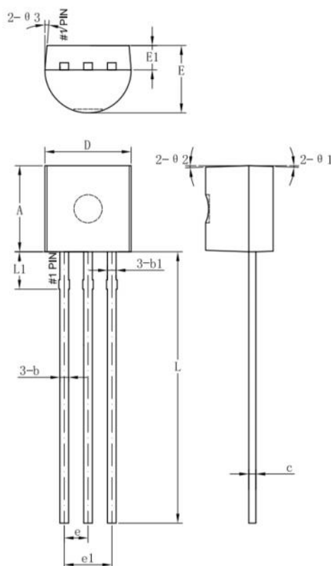
T0-92 外形图
