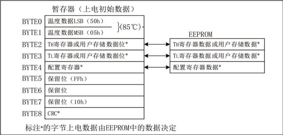
图 2-5 DS18B20-TD存储器映射
