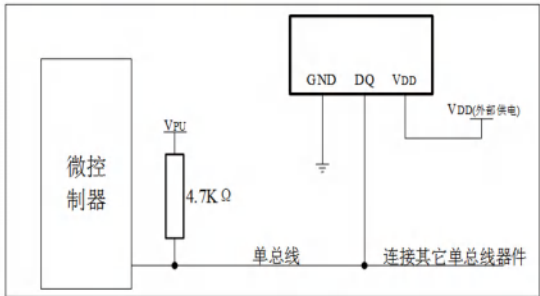
图 2-3 使用外部电源供电
