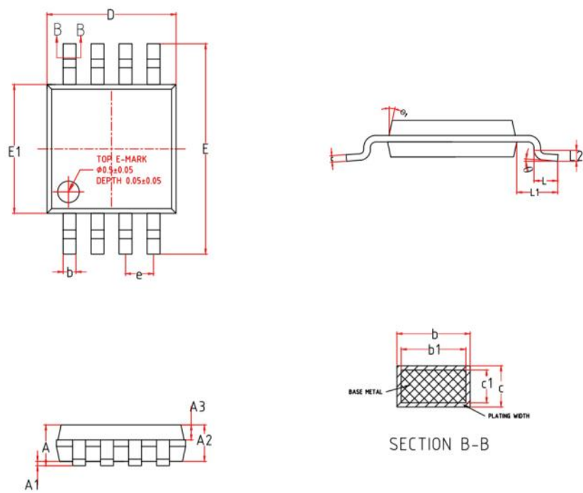
MSOP8 外形图
