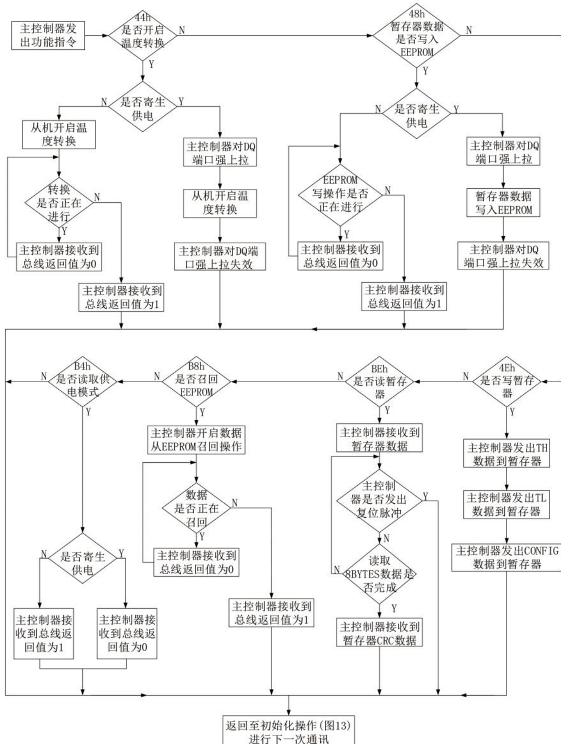
图 2-10 功能指令流程图
