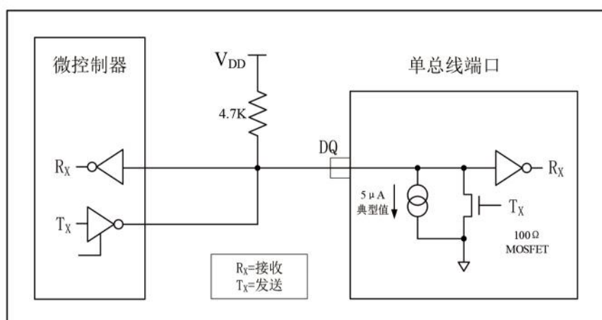
图 2-8 硬件结构
