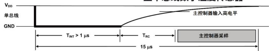
图 2-13 主控制器读取 1 时序
