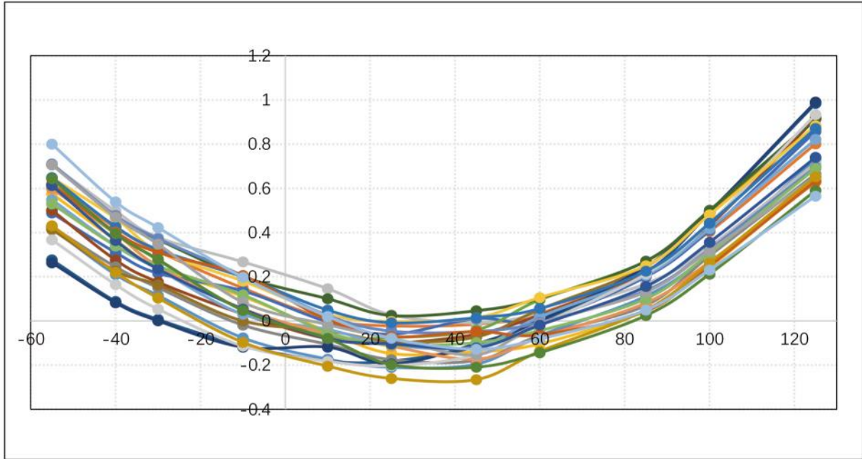
图 1-1 -55~125°C 典型温度误差曲线
