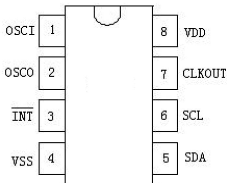
图 3. 引脚图
