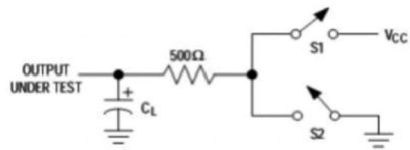
图6驱动时间测试电路
