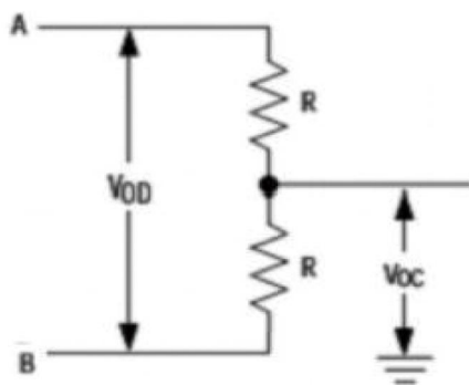
图3 直流驱动测试电路
