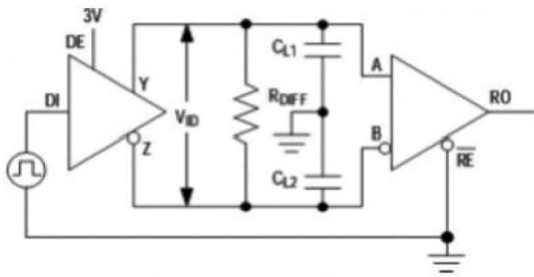
图6驱动时间测试电路
