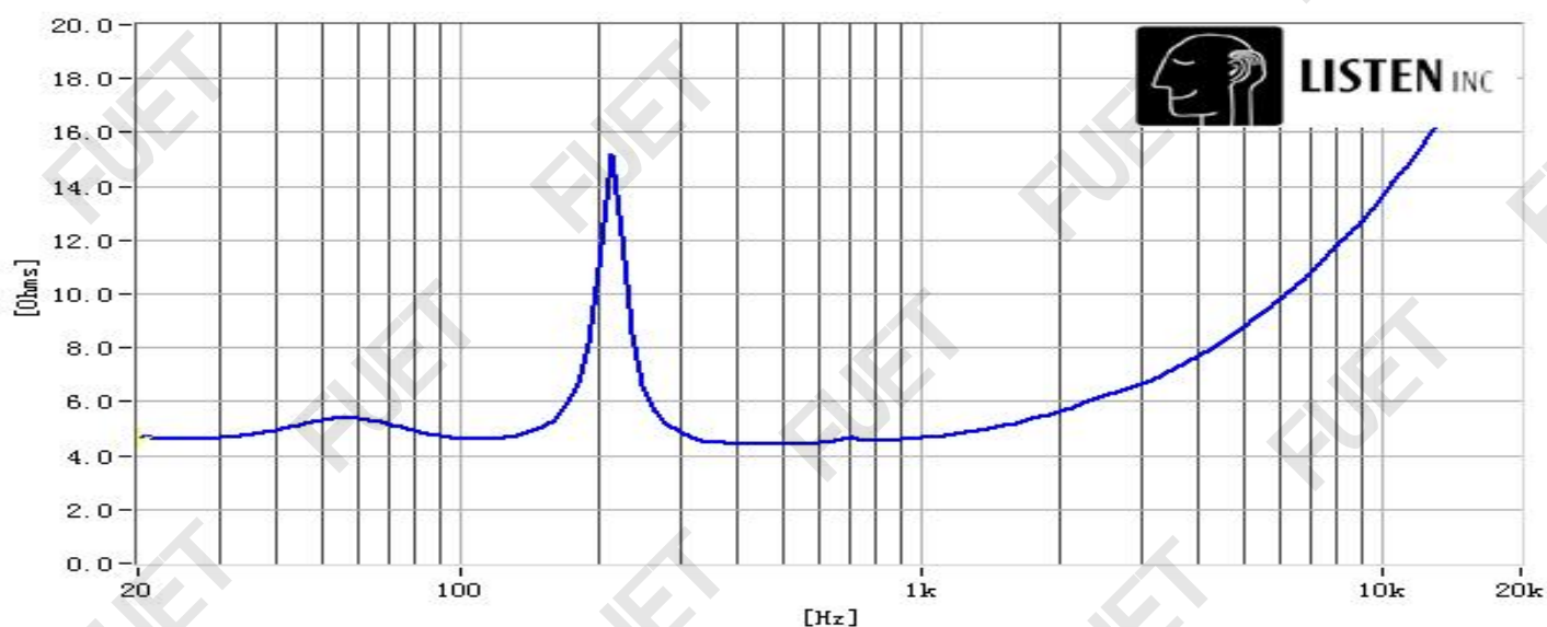
阻抗曲线
