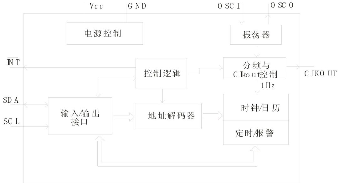
图 2. 方框图
