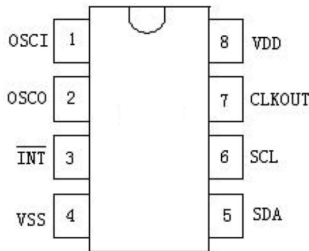
图 3. 引脚图
