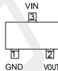
SOT23-3L & SOT23
