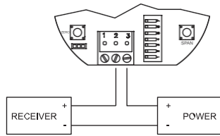
电流输出接线
