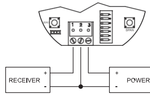
电压输出接线
