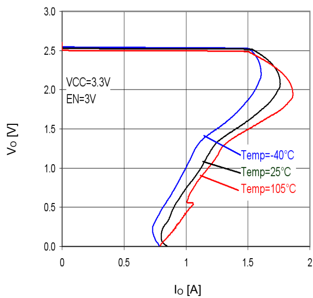
Fig.29 I_o - V_o
