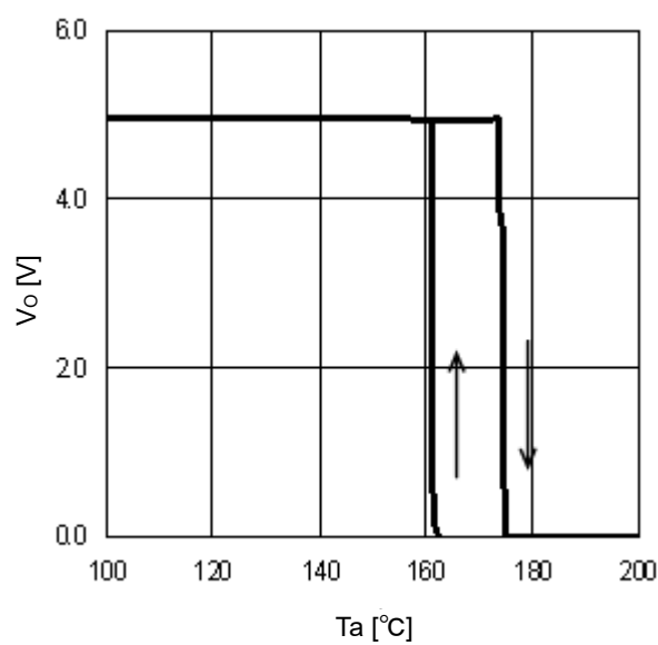
Fig.28 TSD ( I_o=0\text{mA} )
