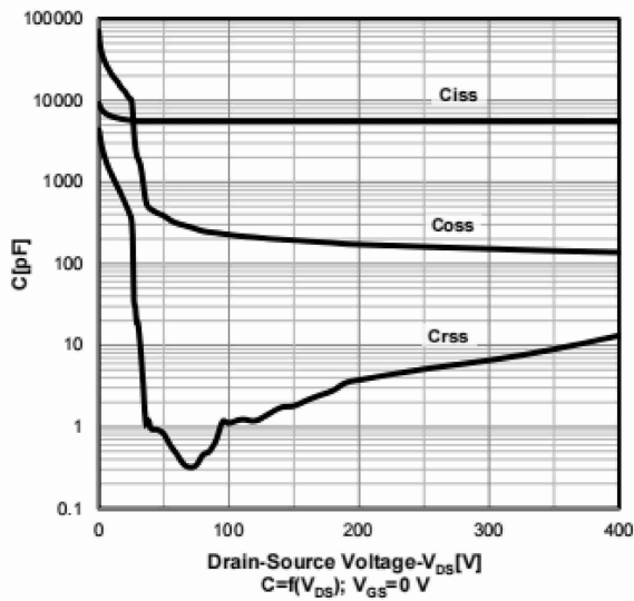
Typ. capacitances
