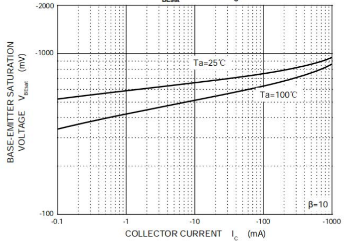
V_{BEsat} — I_c
