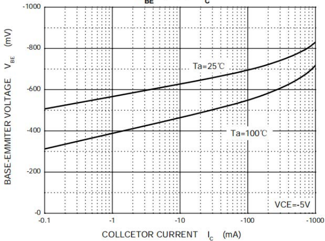
V_{BE} — I_c
