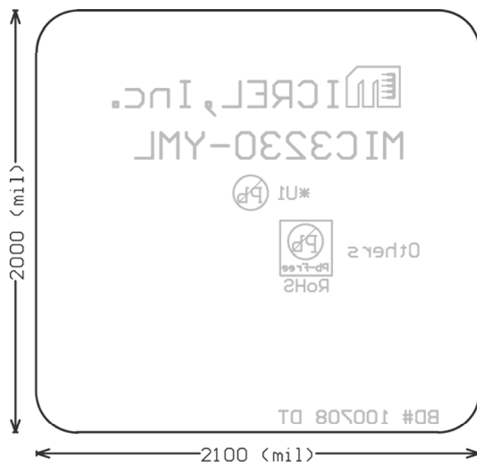
Bottom Layer
