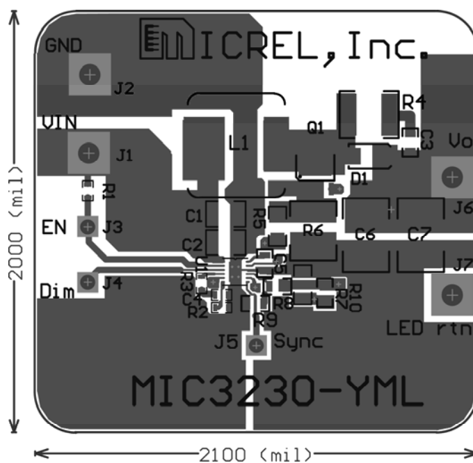
Top Layer
