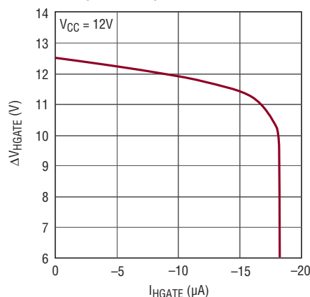
\Delta V_{HGATE} vs I_{HGATE}
