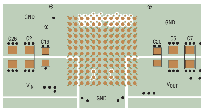
(a) LTM4712 Top Layer
