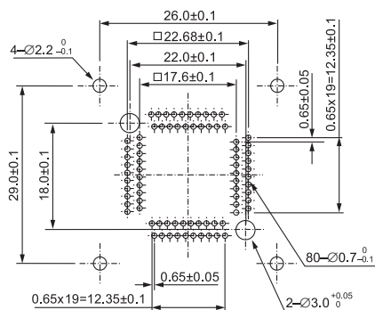
IC51-0804-956-2 (80 Pins)
