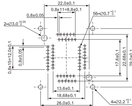
IC51-0564-924 (56 Pins)
