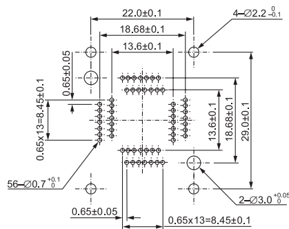
IC51-0564-680 (56 Pins)
