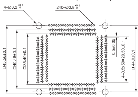
IC51-2404-1655-2 (240 Pins) IC51-2404-1655-3 (240 Pins)
