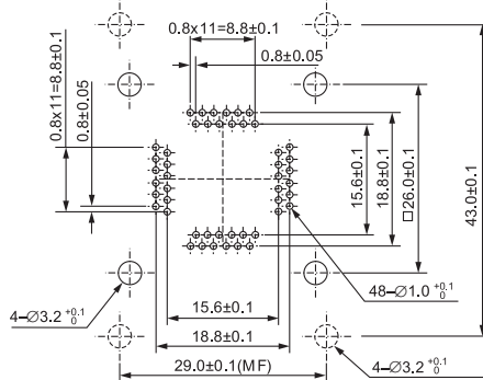
IC51-0484-081 (48 Pins)
