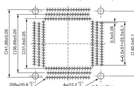
IC51-2084-1052-* 2 (208 Pins)
