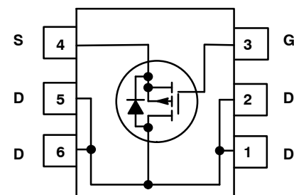
SUPERSOT™-6
