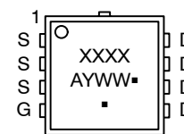
WDFN8 (μ8FL) CASE 511AB
