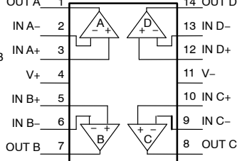
SOIC-14
