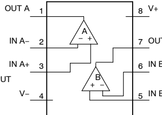
UDFN8/Micro8/SOIC-8
