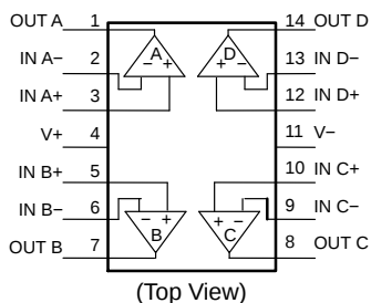
SOIC-14
