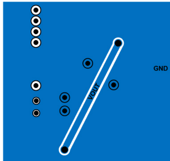
Figure 28. BOTTOM Layer
