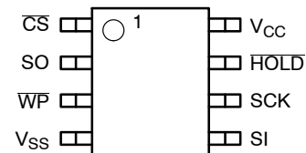
SOIC (V), TSSOP (Y)
