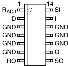
SO-14
