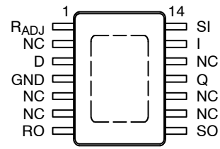
TSSOP-14 EP
