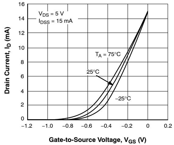
Figure 4. I_D - V_{GS}
