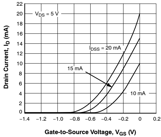
Figure 3. I_D - V_{GS}
