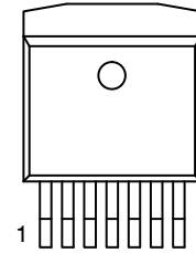
D2PAK-7
